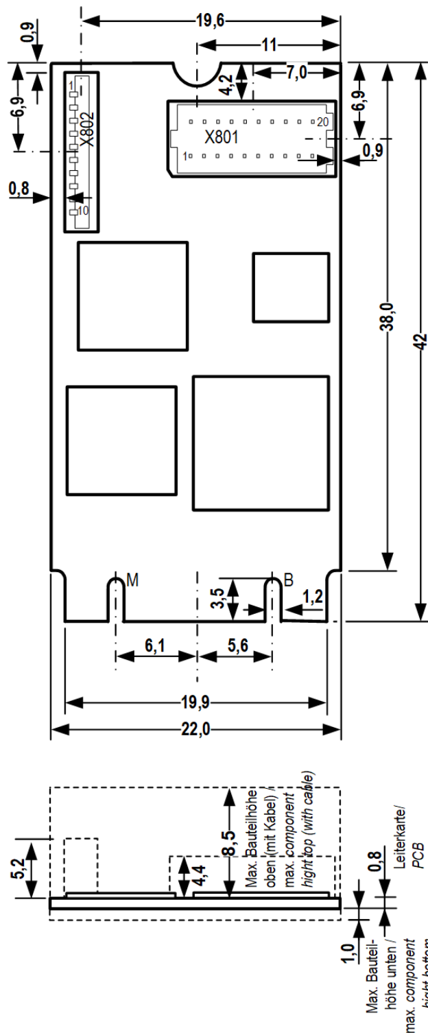
Abbildung 12: Abmessungen CIFS M224290BM (Revision 2)
