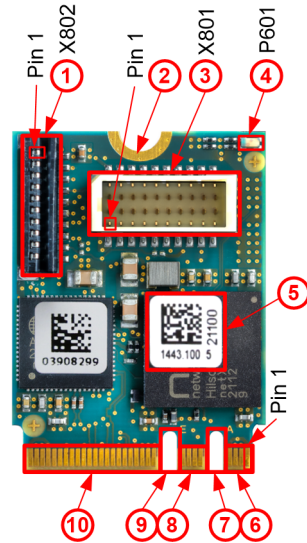
Abbildung 1: Grundkarte CIFX M223090AE (Revision 5)
