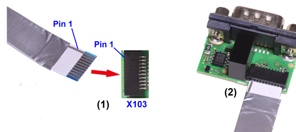
Abbildung 6: Kabel in den Kabelstecker Feldbus X103 auf dem AIFX-V2-CO stecken
