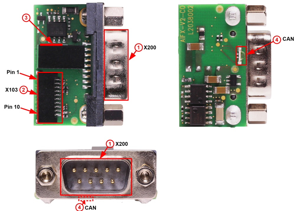
Abbildung 3: Abgesetzte Netzwerkschnittstelle AIFX-V2-CO (Revision 2)
