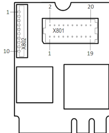
Abbildung 8: Kabelstecker Ethernet X802 (1x10 Pins) auf CIFX M223090AE
