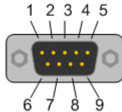
Abbildung 7: CANopen-Schnittstelle (DSub-Stecker, 9-polig), X200
