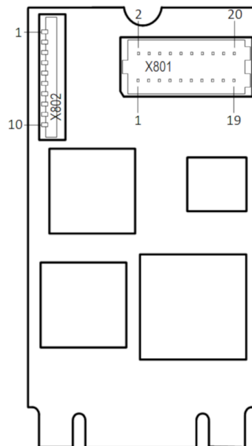
Abbildung 9: Kabelstecker Ethernet X802 (1x10 Pins) auf CIFX M224290BM
