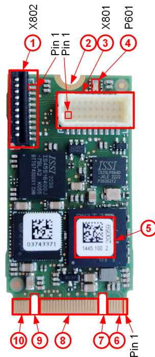
Abbildung 2: Grundkarte CIFX M224290BM (Revision 2)
