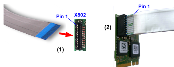
Abbildung 5: Kabel in den Kabelstecker Feldbus auf der Grundkarte stecken, Beispiel M223090AE
